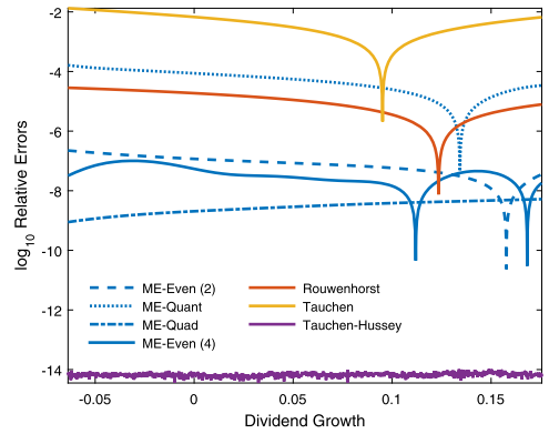
(d) N = 21 .
