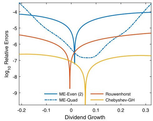
(d) \rho = 0.99 .
